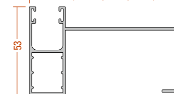
AL HSLA-25
