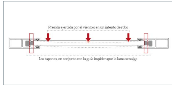
Esquema de funcionamiento del sistema Extreme de Persax.
