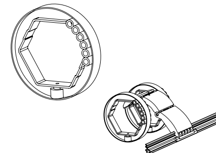
111531 ANILLO TIRANTE SEGURIDAD BLOQUEO E60 111846 ANILLO TIRANTE SEGURIDAD BLOQUEO E70 BLOCK SECURITY SPRING RING (S60-S70) ANNEAU ATTACHE SÉCURITÉ BLOCAGE (A60-A70)
