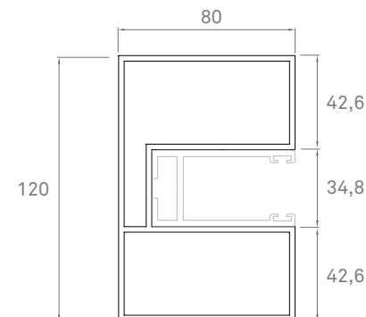
■ 308219 GUÍA AL PREMARCO 120X80 MM DOBLE TAQUILLA GUIDE TO PRE-FRAME 120 X 80 MM DOUBLE LOCKER GUIDE POUR LE PRÉCADRE 120 X 80 MM DOUBLE CASIER
